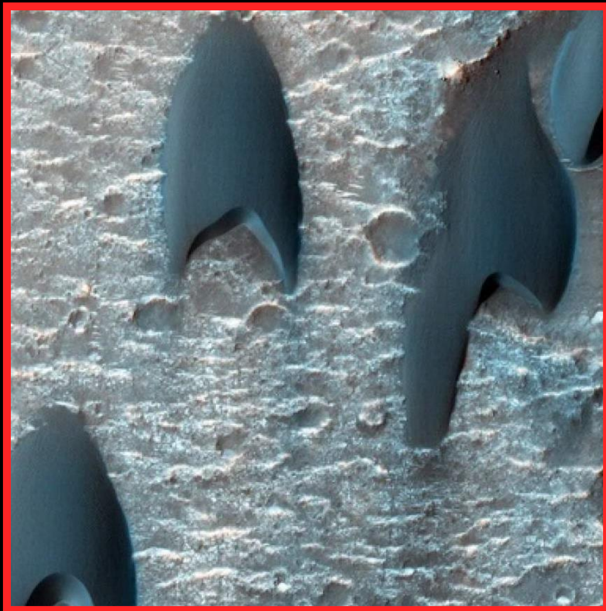
Barchan dunes, Mawrth Valley
