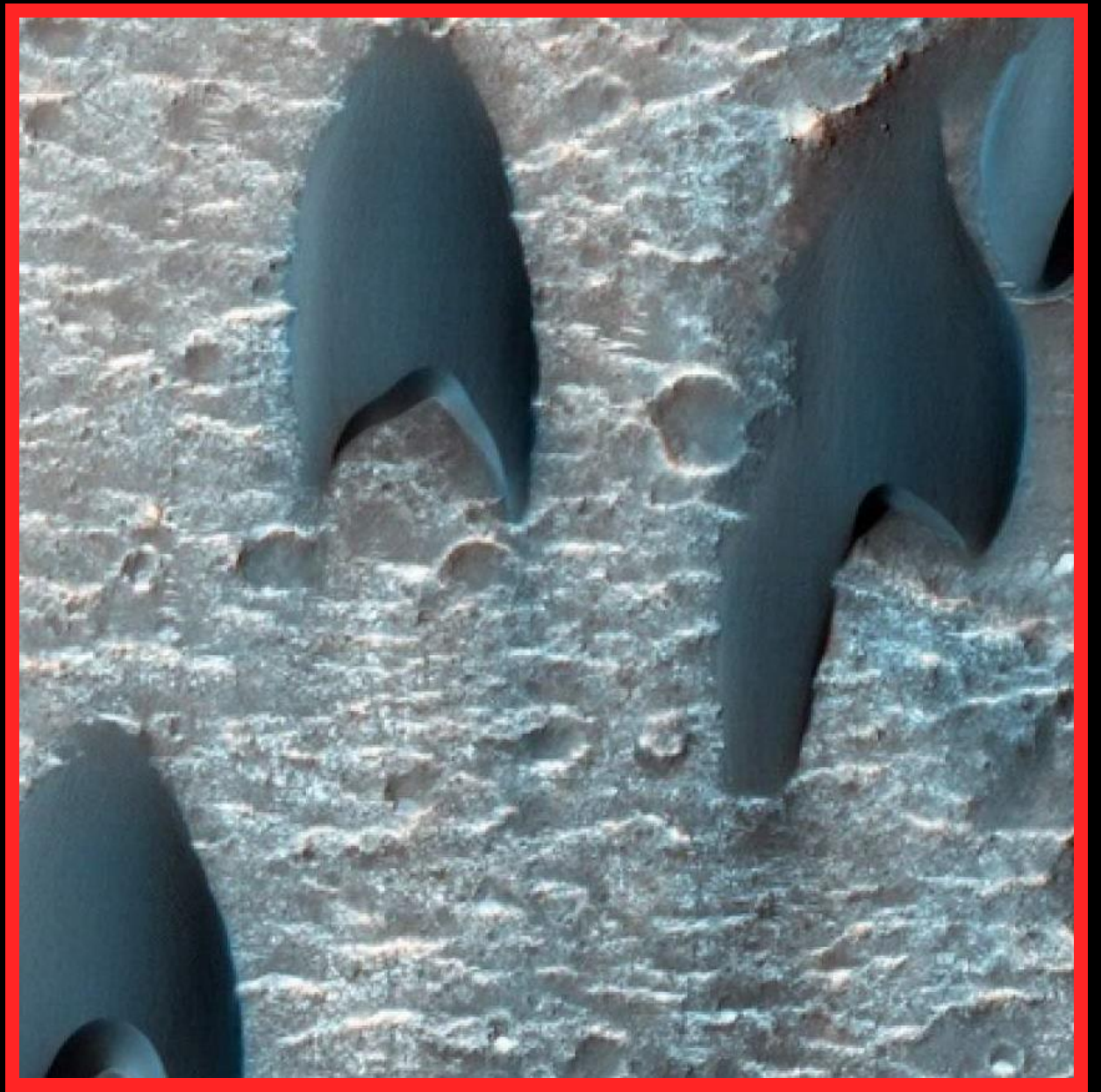
Barchan dunes, Mawrth Va
